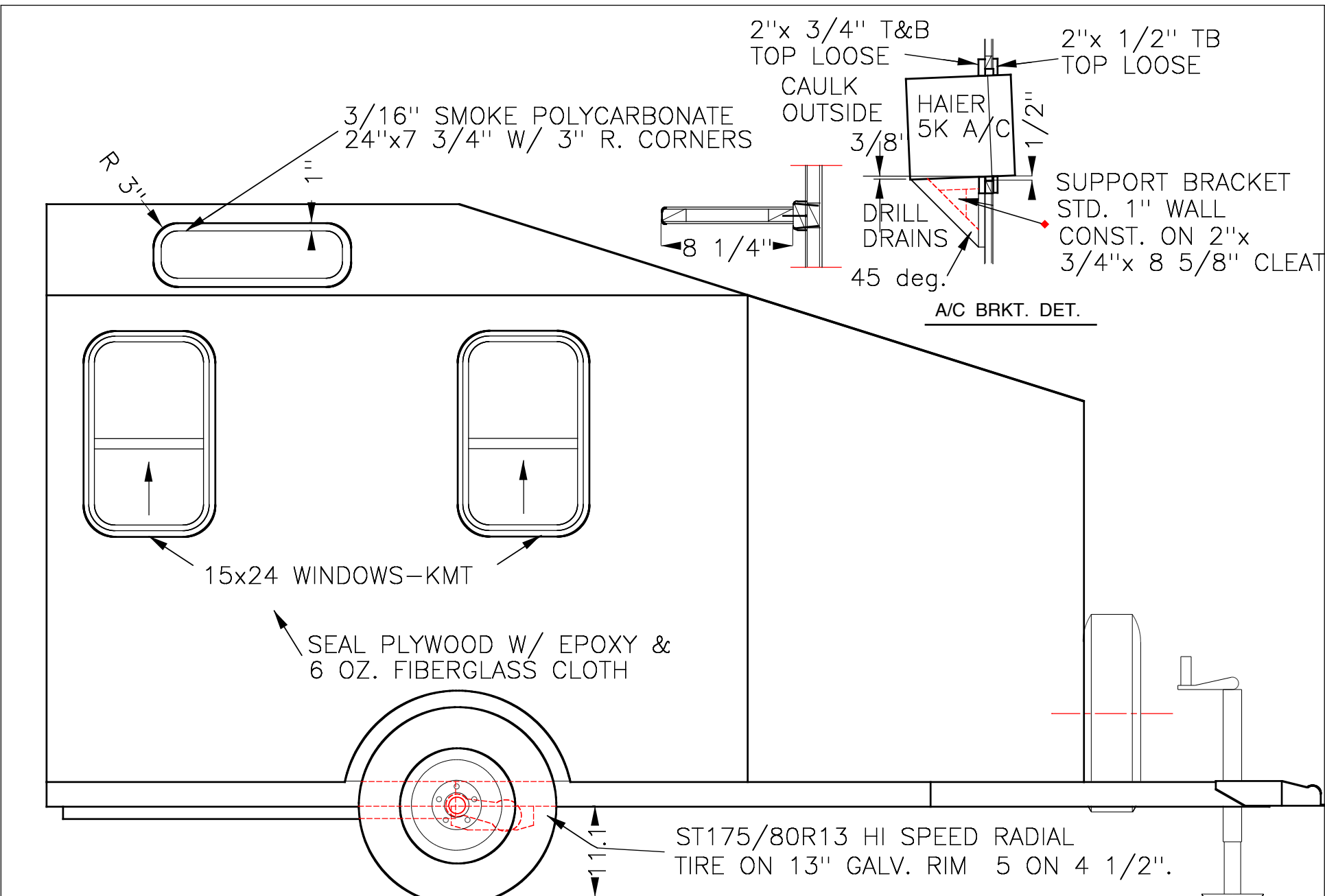
RIGHT EXT. ELEVATION
